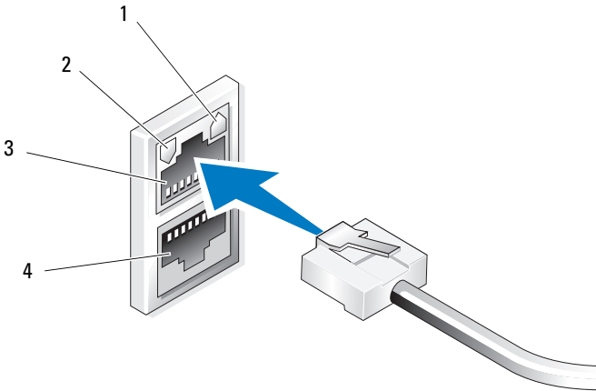
그림 1-2. NIC 커넥터
